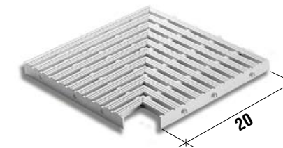
A003637 Angolo per griglia parallela Gr20
