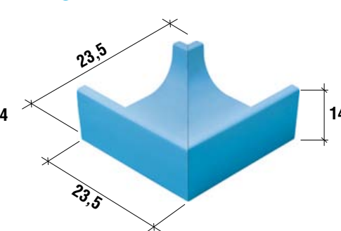
4 Canale basso angolo esterno
